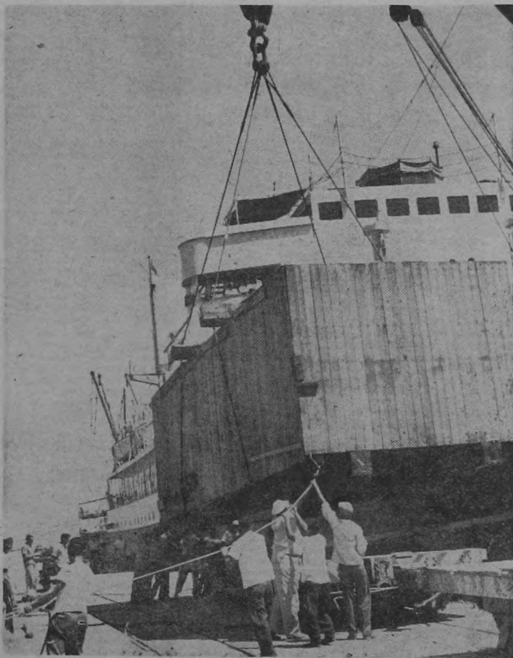
La valiosísima colaboración del Jefe de Muelle, Coronel Lisímaco Azofeifa, fue indispensable para la rapidez en la descarga y colocación de la maquinaria en los carros del Ferrocarril Eléctrico al Pacífico.
